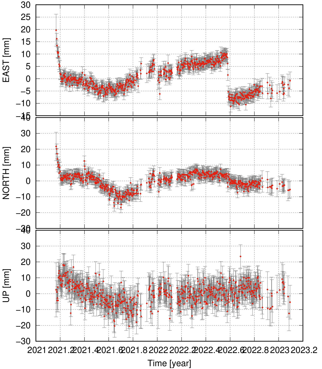
AFST residual time series
