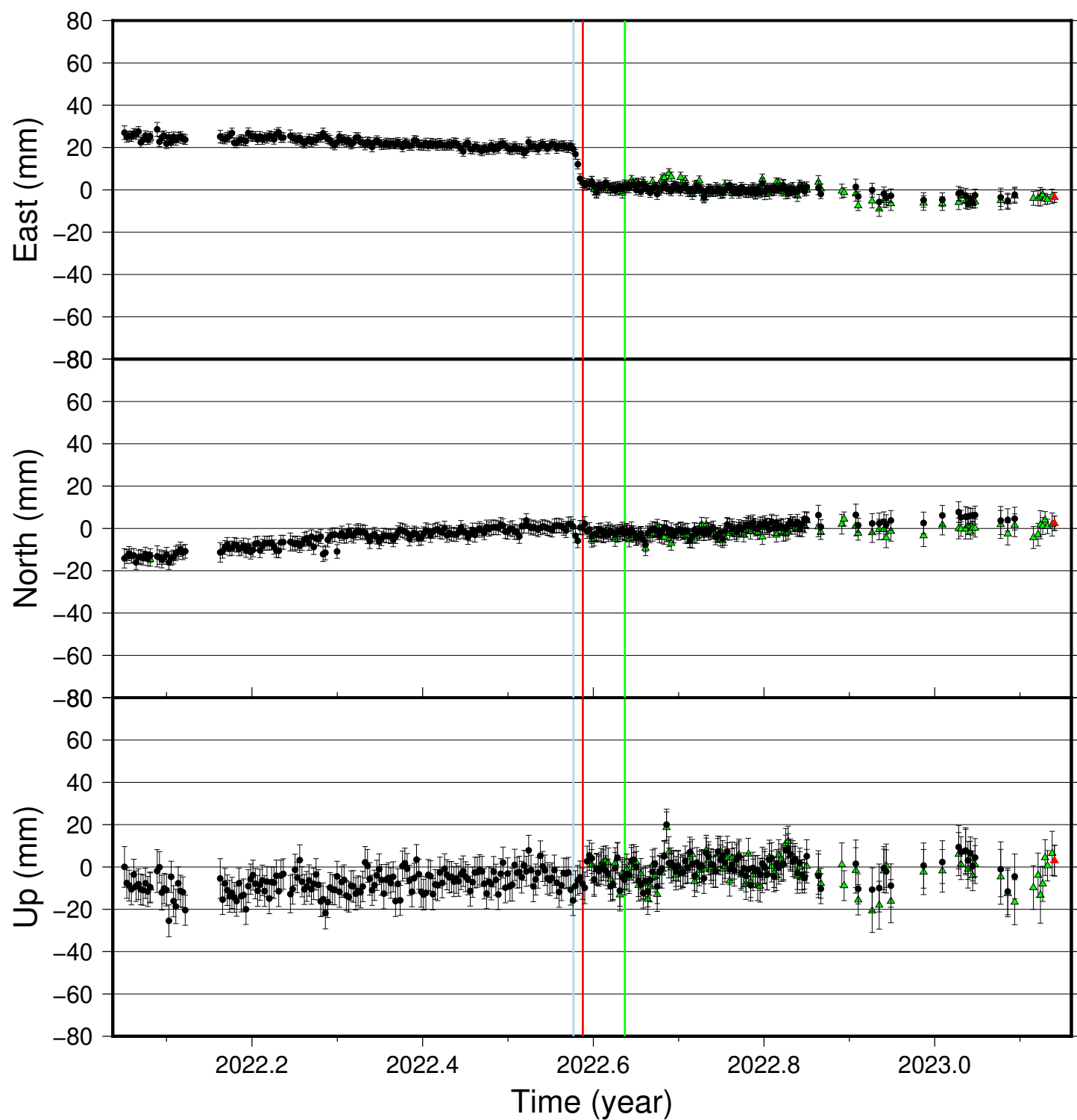
AFST time series (IGS 2014), last 400 days
